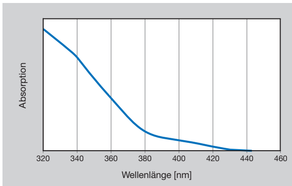
Absorptionsspektrum des Photoiniators (Wellenlängenbereich von 320 – 450 nm) der UV- und lichthärtenden DELO PHOTOBOND in einer Acrylatmatrix
