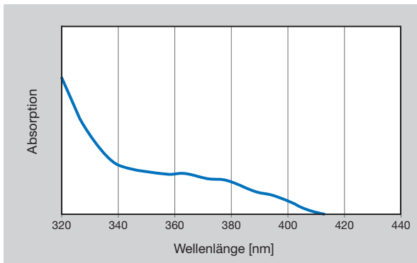
Absorptionsspektrum des Photoiniators (Wellenlängenbereich von 320 – 420 nm) der UV- und lichthärtenden DELO PHOTOBOND in einer Acrylatmatrix
