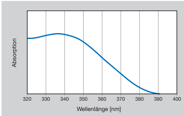
Absorptionsspektrum des Photoiniators (Wellenlängenbereich von 320 – 400 nm) der UV-härtenden DELO PHOTOBOND in einer Acrylatmatrix
