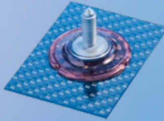
Kleben von strukturellen Verbindungselementen (ONSERT®)
