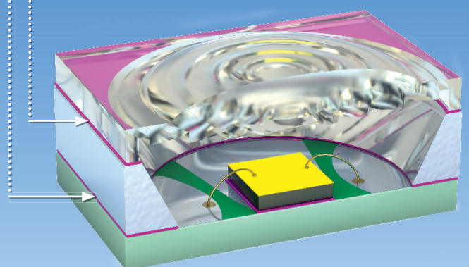
Optical Packaging – Verkleben Gehäuse / Leiterplatte sowie Glasabdeckung / Gehäuse
